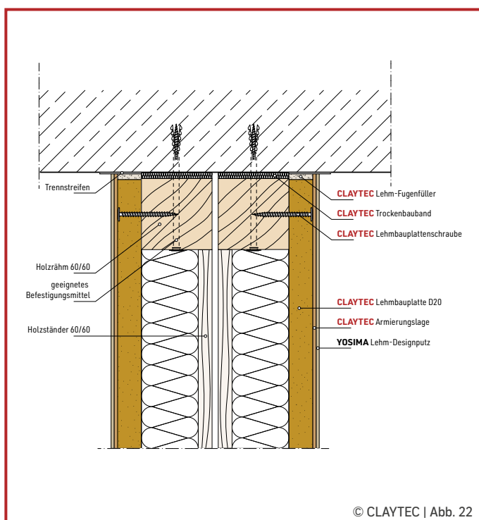
Holzkonstruktion Doppelständer Anschluss an Massivdecke
