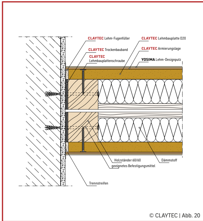
Holzkonstruktion Doppelständer Anschluss an Massivwand
