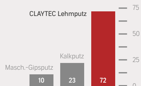
Luftfeuchteaufnahme nach 12 h in g/m 2 (DIN 18947)
